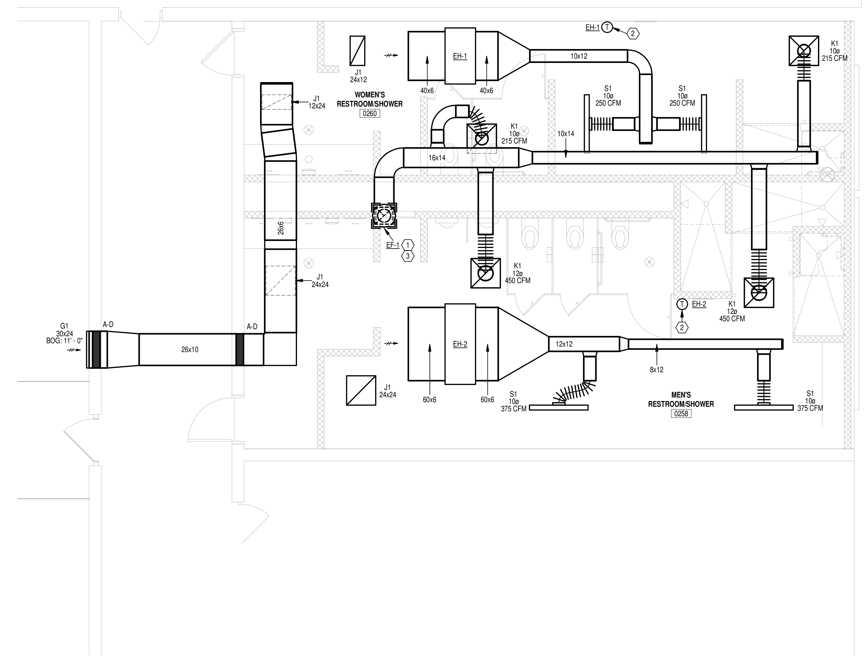
1 - HVAC - NEW SCALE: 1/4" = 1'-0"
